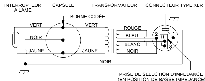
BRANCHEMENTS INTERNES
