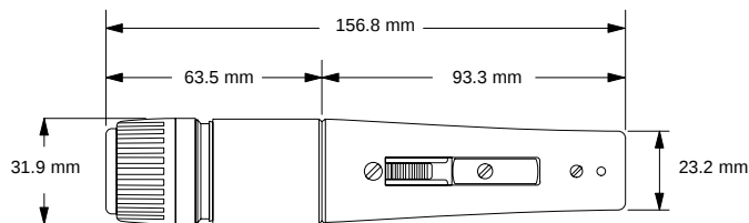
DIMENSIONI COMPLESSIVE
