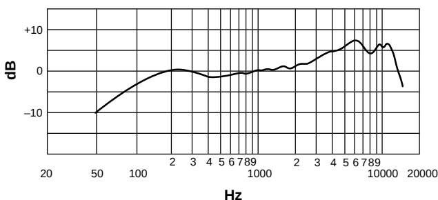
RESPUESTA DE FRECUENCIA TÍPICA
