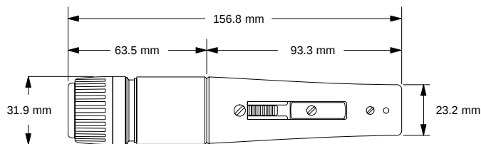
GESAMTABMESSUNGEN
