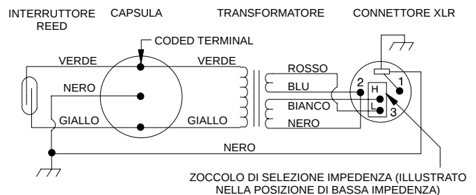
CONNESSIONI INTERNE
