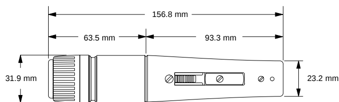
DIMENSIONES GENERALES
