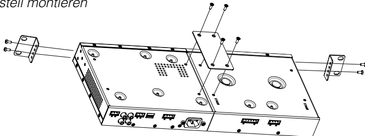
Abbildung 2.2.3 Verstärker und CST-2120 Transformermodule auf Gestell montieren
