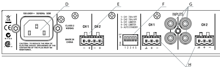
Abbildung 3.3 Rückansicht
