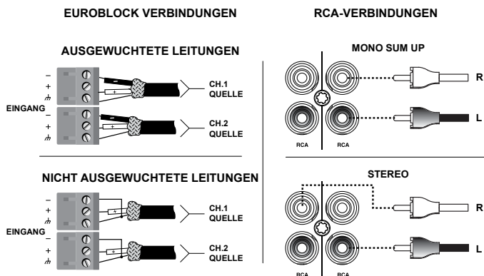
Abbildung 2.4 Eingangsverdrahtung
