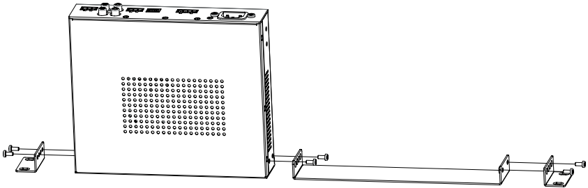
Abbildung 2.2.4 Gestellmontage einzelner Verstärker
